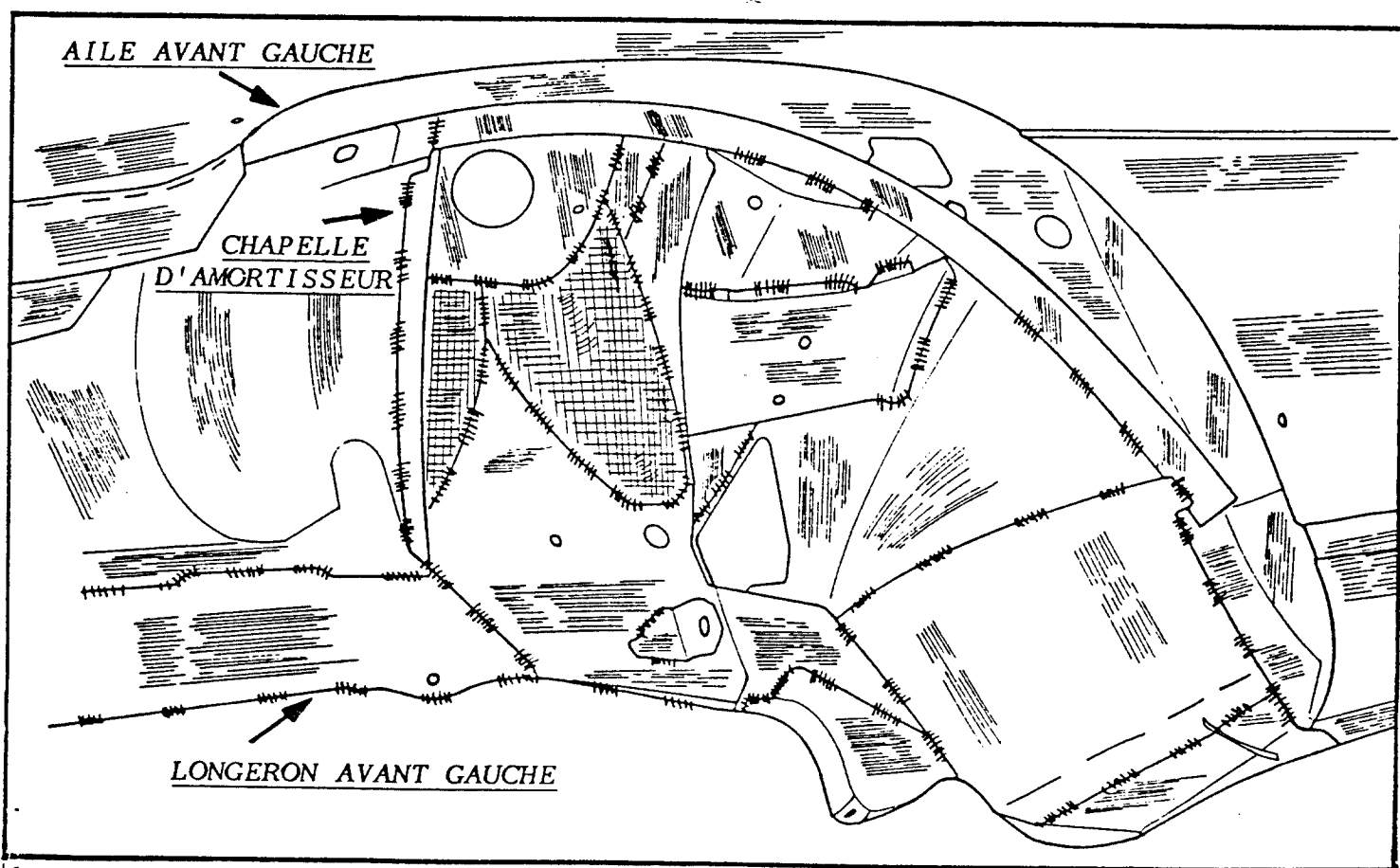
LIAISON CHAPELLE D'AMORTISSEUR AVANT / LONGERONS AVANT DROIT ET GAUCHE (VUE DE DESSOUS)
