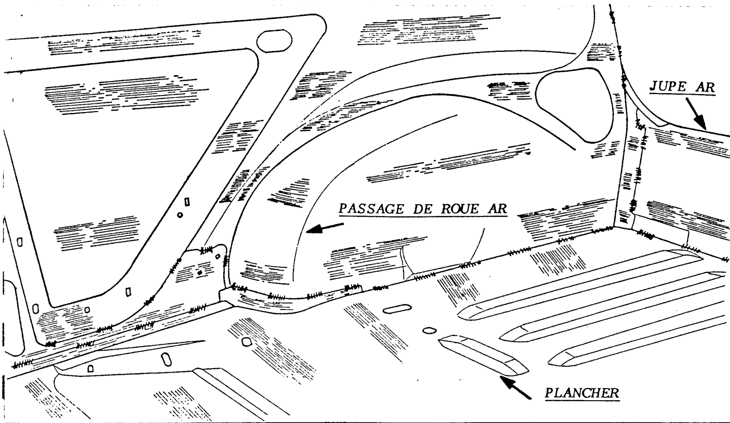
LIAISON PLANCHER ARRIERE / DEMI-BLOC ARRIERE DROIT ET GAUCHE
