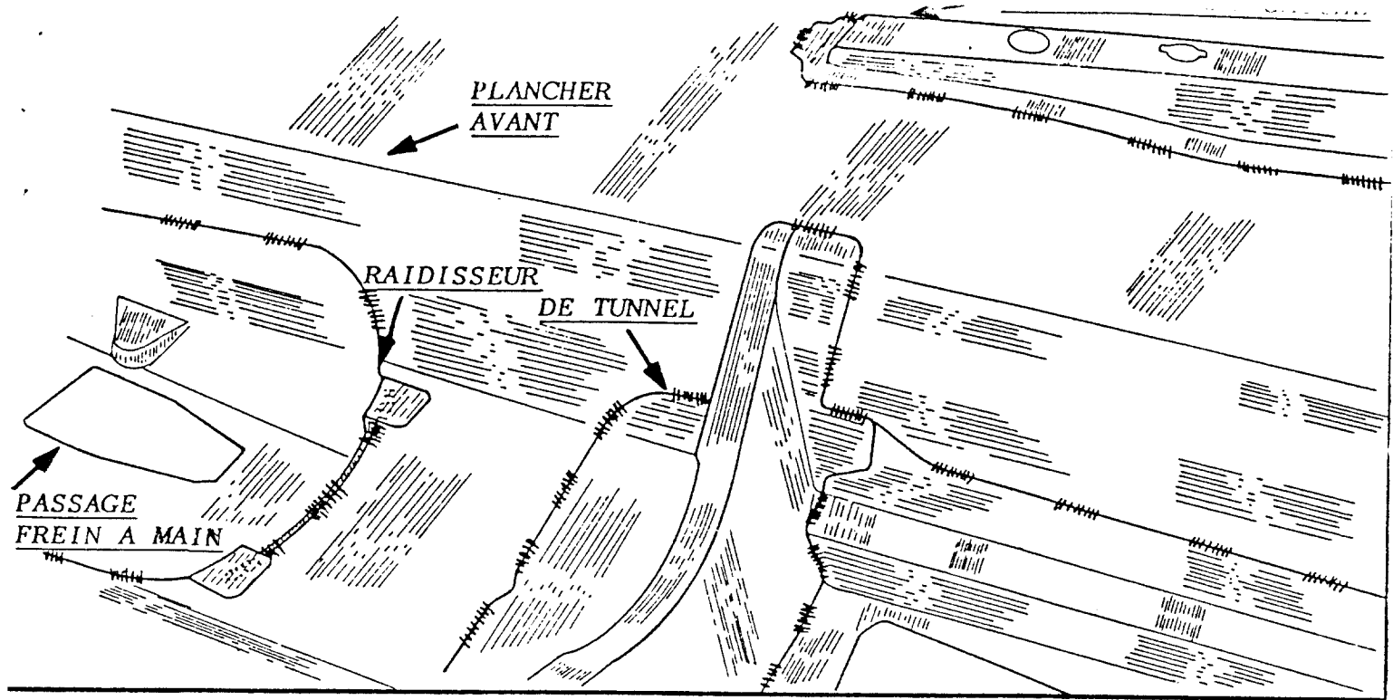
LIAISON PLANCHER AVANT / LONGERONS AVANT DROIT ET GAUCHE + RAIDISSEUR DE TUNNEL (VUE DE DESSOUS)
