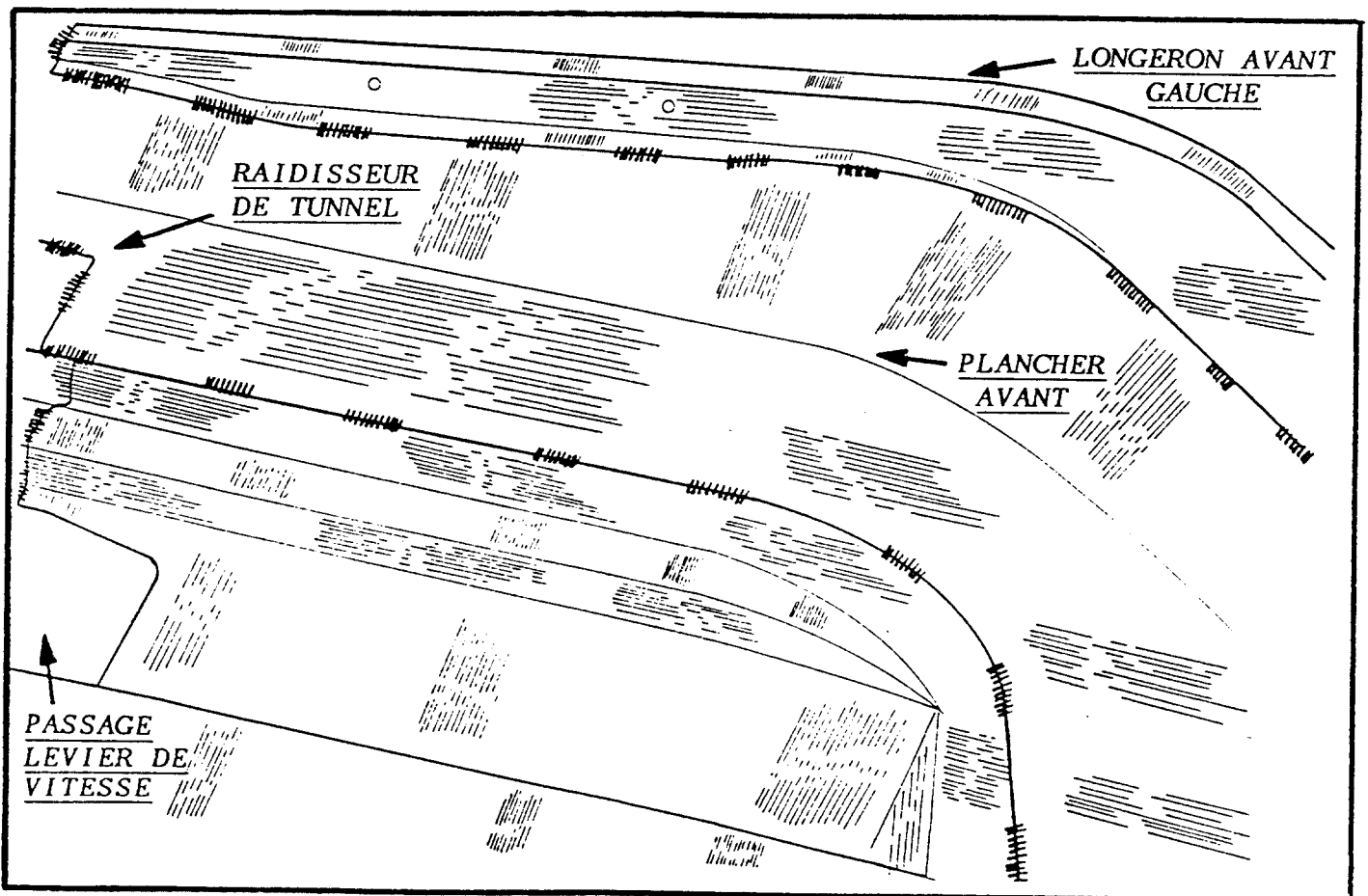
LIAISON PLANCHER AVANT / LONGERONS AVANT DROIT ET GAUCHE + RAIDISSEUR DE TUNNEL
