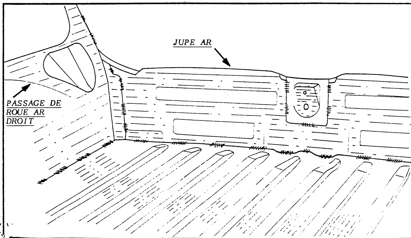
LIAISON PLANCHER ARRIERE / JUPE ARRIERE
