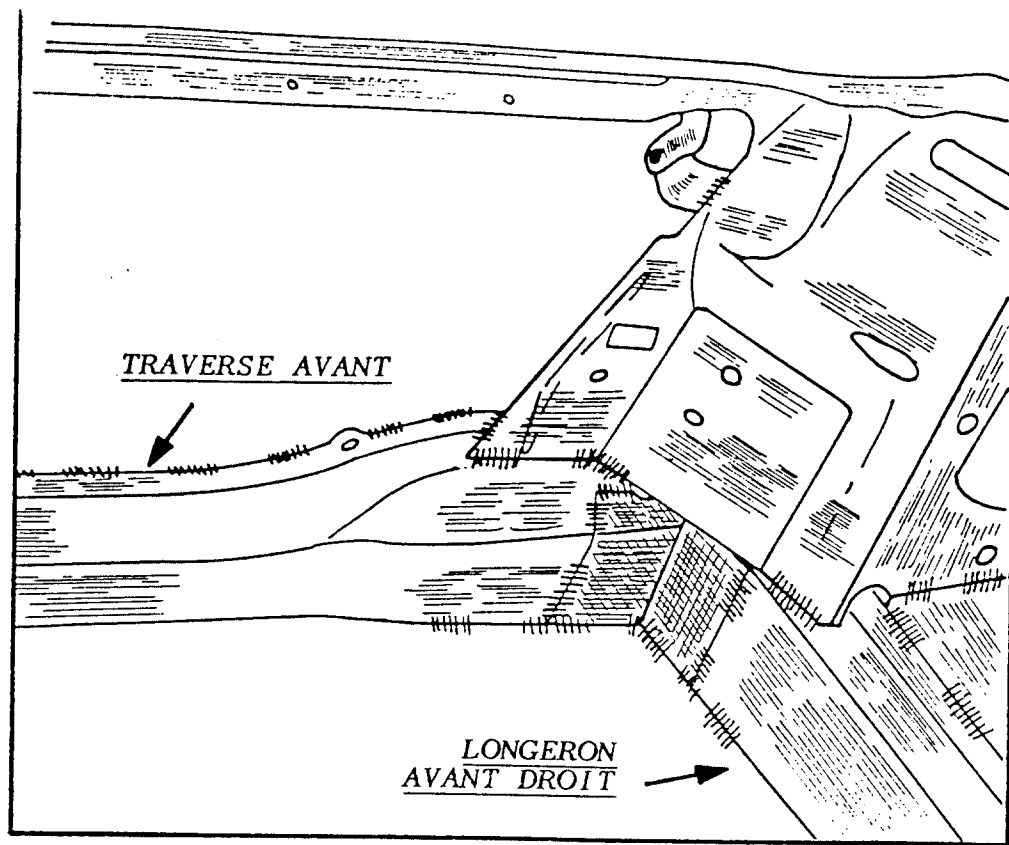
LIAISON UNIT AVANT / LONGERONS AVANT DROIT ET GAUCHE (VUE INTERIEURE)
