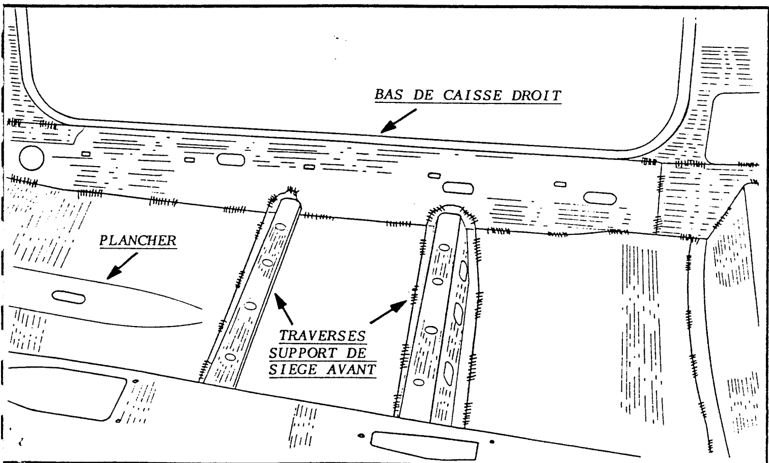
LIAISON PLANCHER AVANT / BAS DE CAISSE DROIT ET GAUCHE
